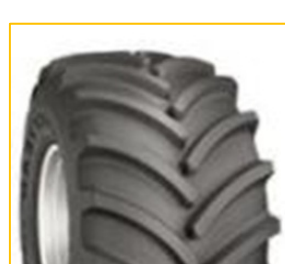
guma+felga: 677229/1 280-70 R18 Širina: 280 mm Visina: 70% širine (19,6 cm) Felga premer: 18" (45,75 cm)
